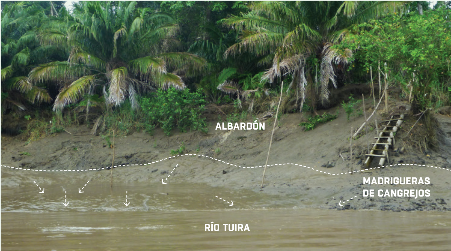
FIGURA 2: Vista del albardón desde el cauce del río Tuira. La línea punteada indica la descarga subterránea desde el albardón hacia el río durante marea baja (Fuente: Carol et al. 2020).
